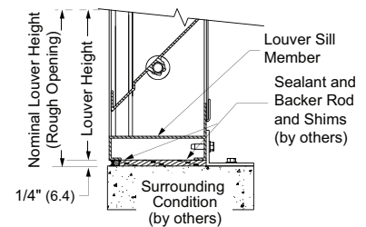
Fig. 2.4 Sill
