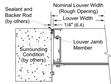
Fig. 2.3 Jamb
