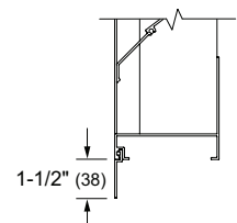
Flange Frame
